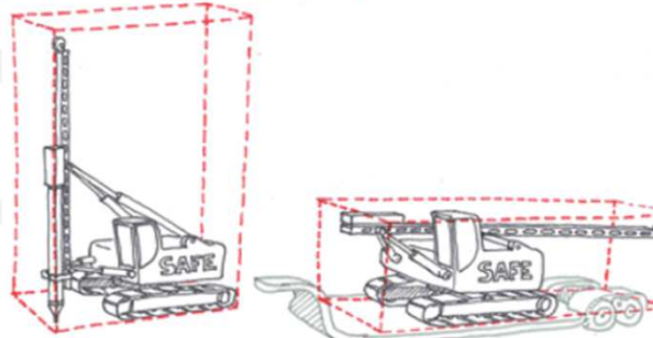
En påkran är en typisk stor grundläggningsmaskin (se bild ...).
